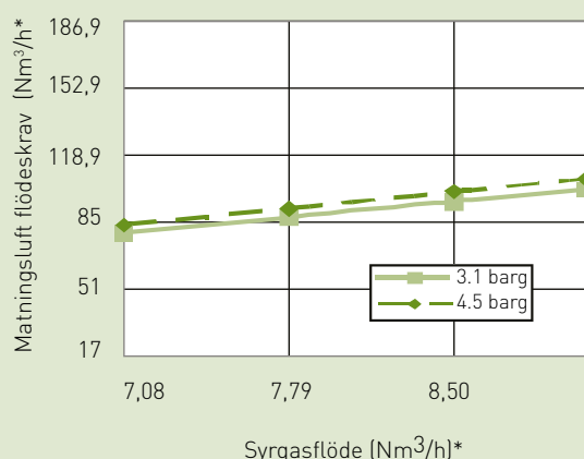
Modell AS-G syrgasgenerator matningsluftskrav** (93% nominell syrgas)
