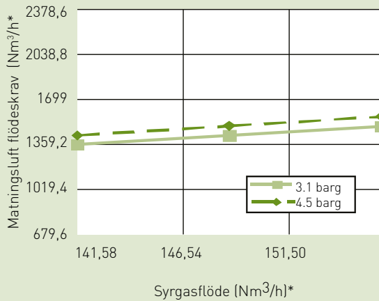
Modell AS-Z syrgasgenerator matningsluftskrav** (93% nominell syrgas)
