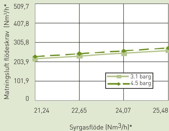
Model AS-K syrgasgenerator matningsluftskrav** (93% nominell syrgas)
