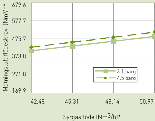
Modell AS-N o syrgasgenerator matningsluftskrav** (93% nominell syrgas)
